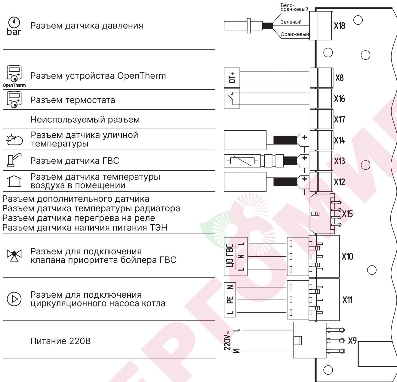
Рис.4 Схема подключения датчиков «ZOTA X-Line100E».
