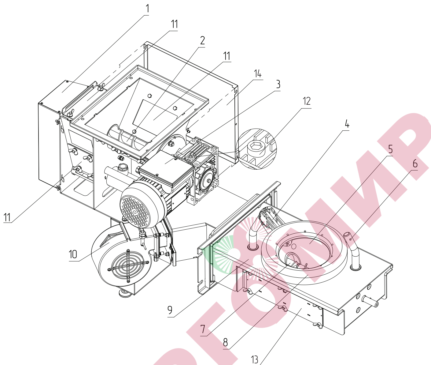
Рис.3 Пеллетная горелка котла ZOTA Pellet Black
