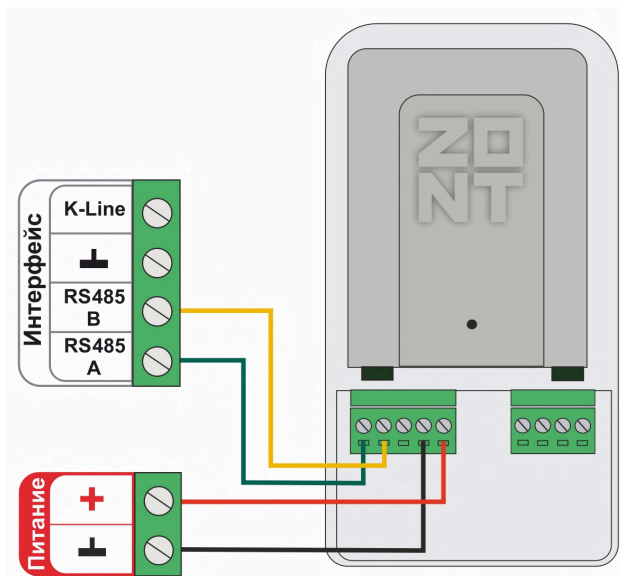
Схема подключения внешнего адаптера цифровой шины ECO по RS-485 :
