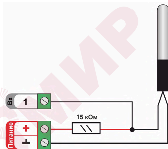
Схема подключения датчика NTC-10 к универсальному входу.
