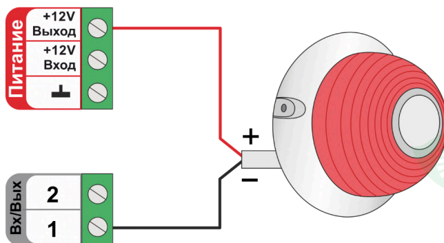
Схема подключения к выходу ОК:
