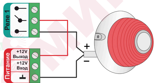
Схема подключения к релейному выходу:
