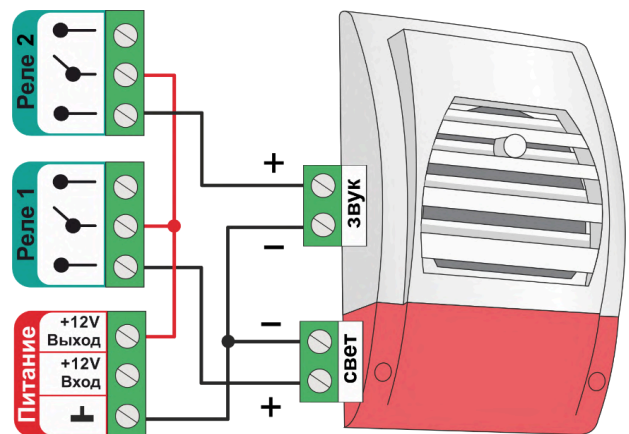
Схема подключения к релейному выходу
