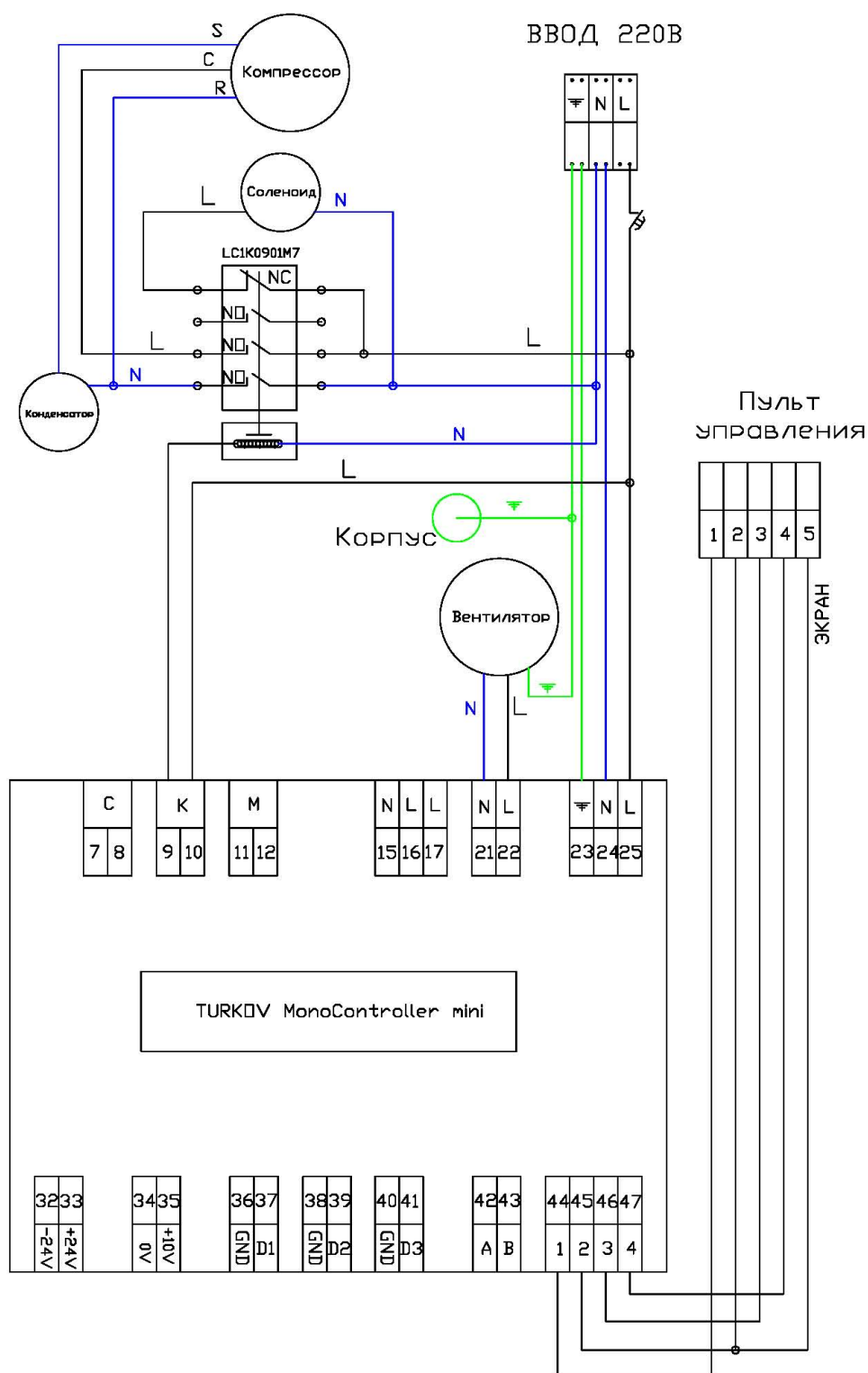
Электрическая схема OS-800
