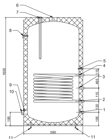
Рис. 3. Размеры SWH-2110-300
