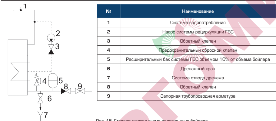
Рис. 15. Гидравлическая схема подключения бойлера
