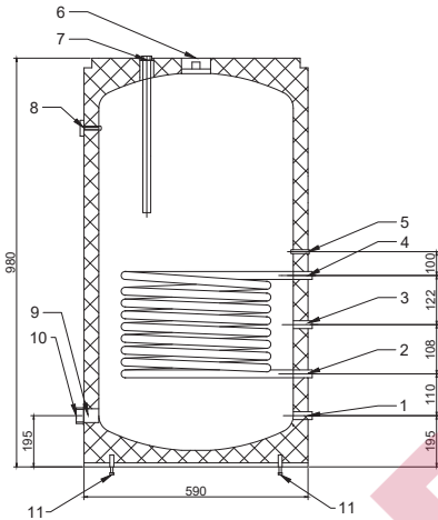
Рис. 1. Размеры SWH-2110-150
