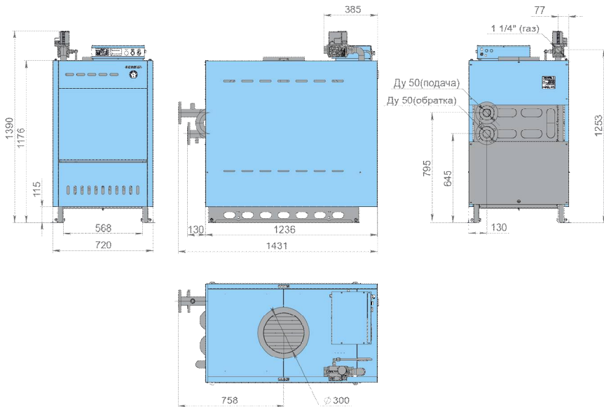
Рисунок 2. Габаритно-присоединительные размеры котла RSA200
