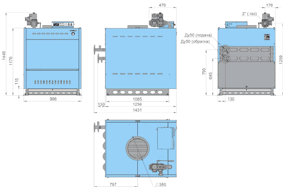
Рисунок 4. Габаритно-присоединительные размеры котла RSA300
