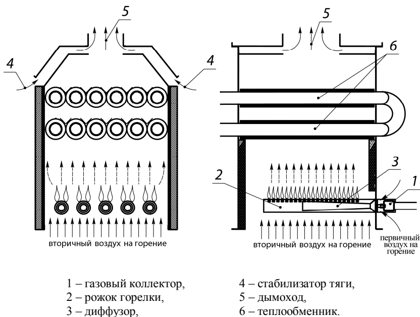
Рисунок 9. Принцип работы
