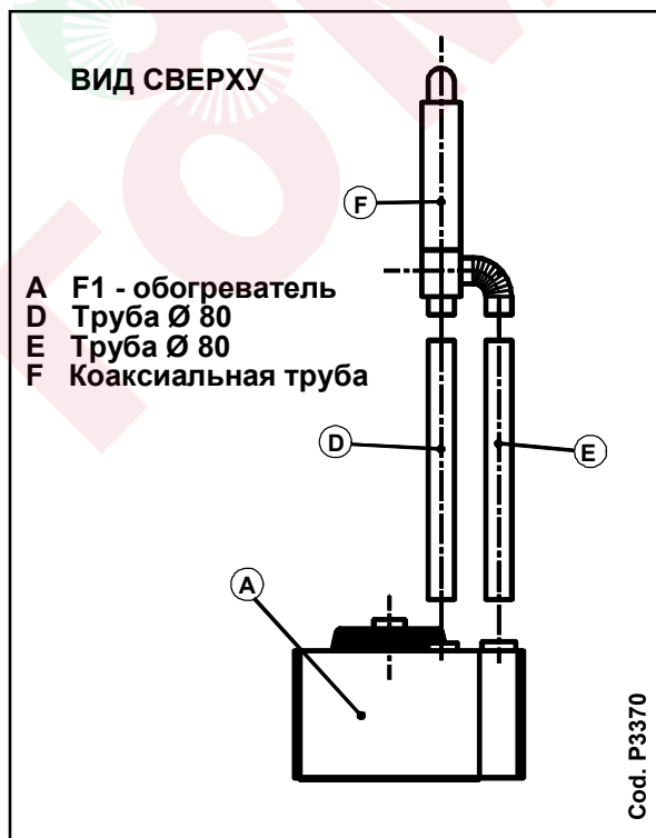
Рисунок 9 С13 УСТАНОВКА С КОАКСИАЛЬНЫМ ТРУБОПРОВОДОМ СТЕНЫ
