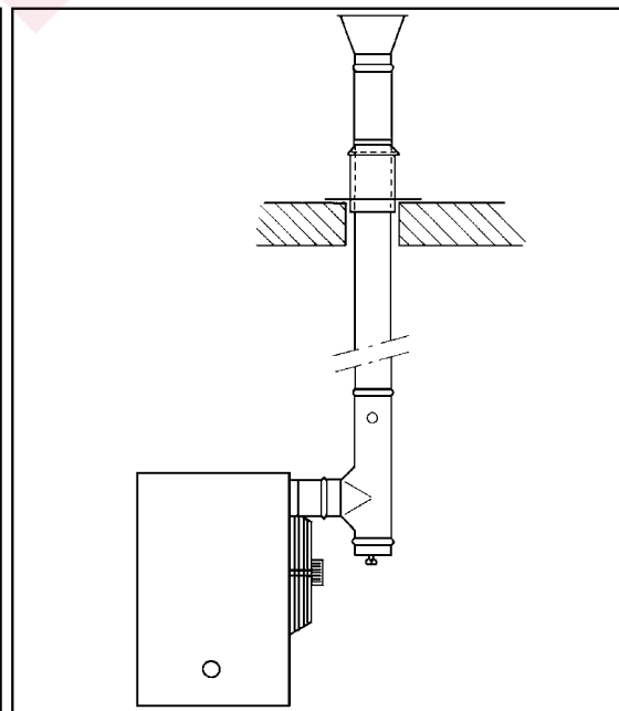
Рисунок 7 - ТИП УСТАНОВКИ В23(КРОВЛЯ)
