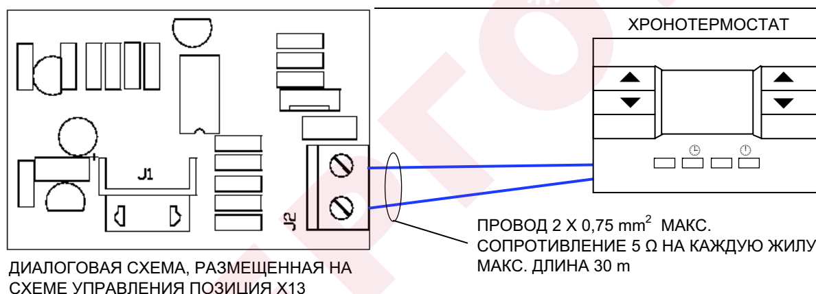
Рисунок 30 – Соединение хронотермостата и диалоговой схемы
