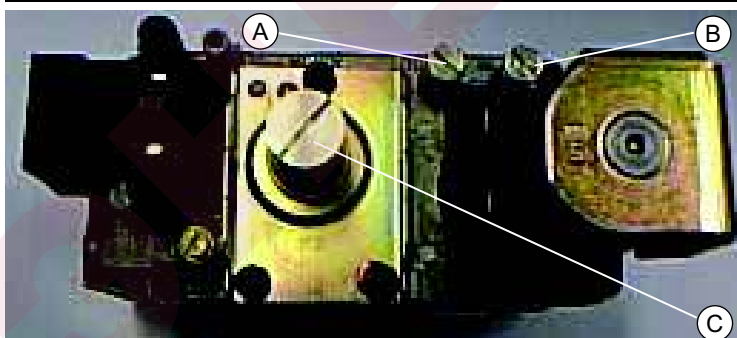
Рисунок 33 – Клапан "Sit 822 Novamix"
