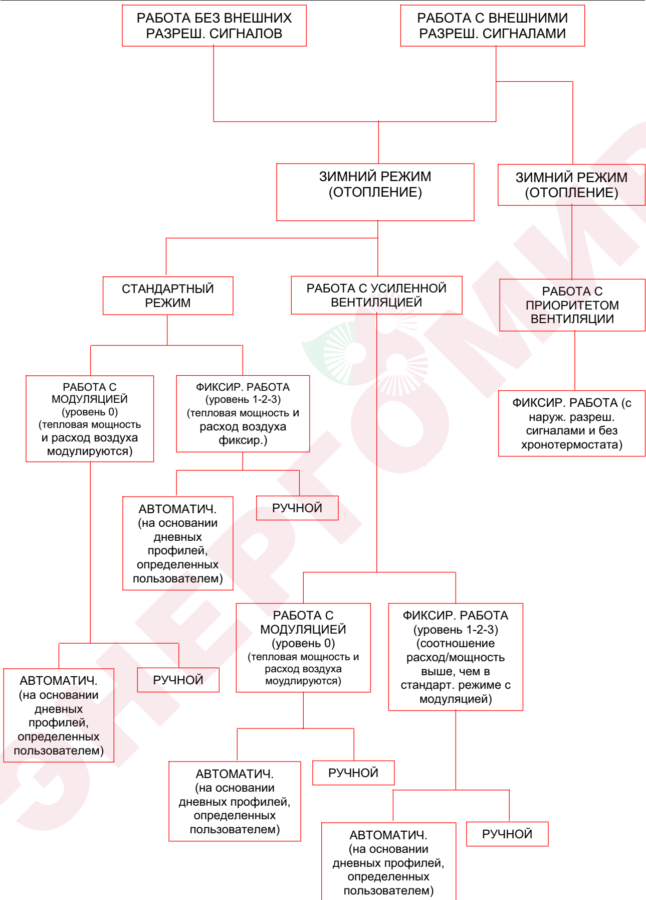
Рисунок 12 – ЗИМНИЙ РЕЖИМ
