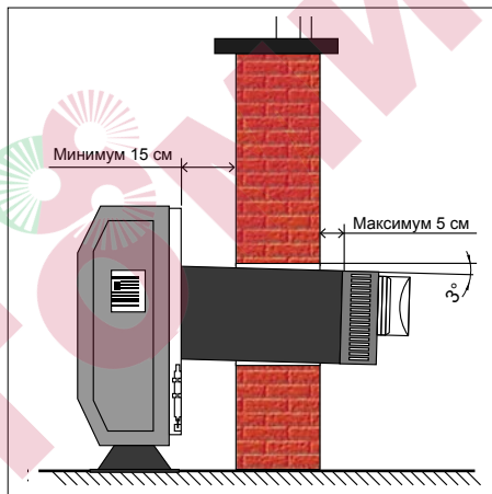
Рисунок 1Б: Расстояние задней панели от стены (модель NHS).
