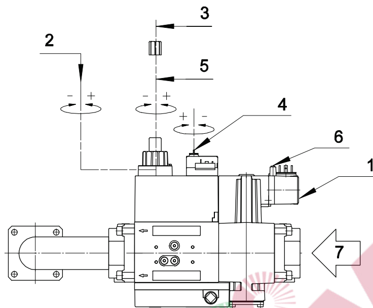
Fig. 16 DUNGS MB-DLE
