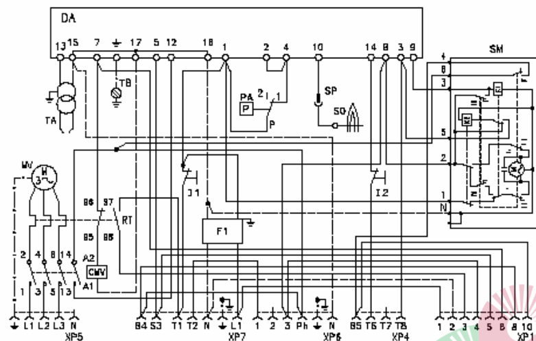
СХЕМА (A) Горелка RS 50 (трехфазная)
