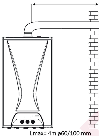
а) Пример дымохода с использованием одного 90^\circ отвода.
