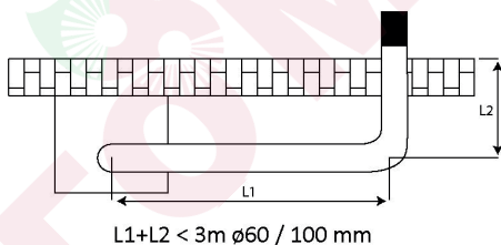
б) Пример дымохода с использованием двух 90^\circ отводов.
