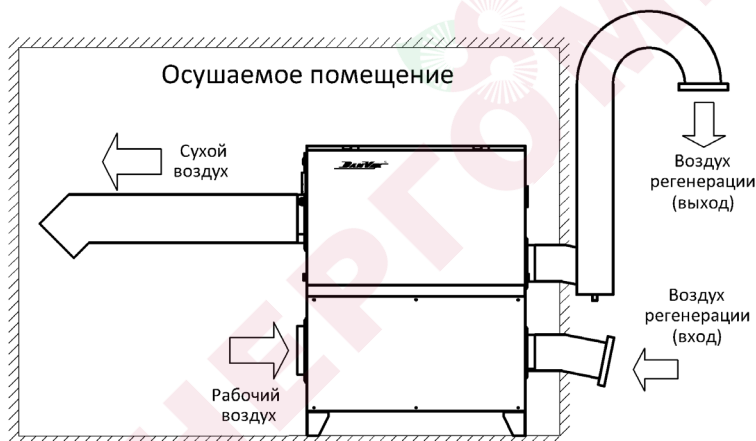
Схема внутренней установки
