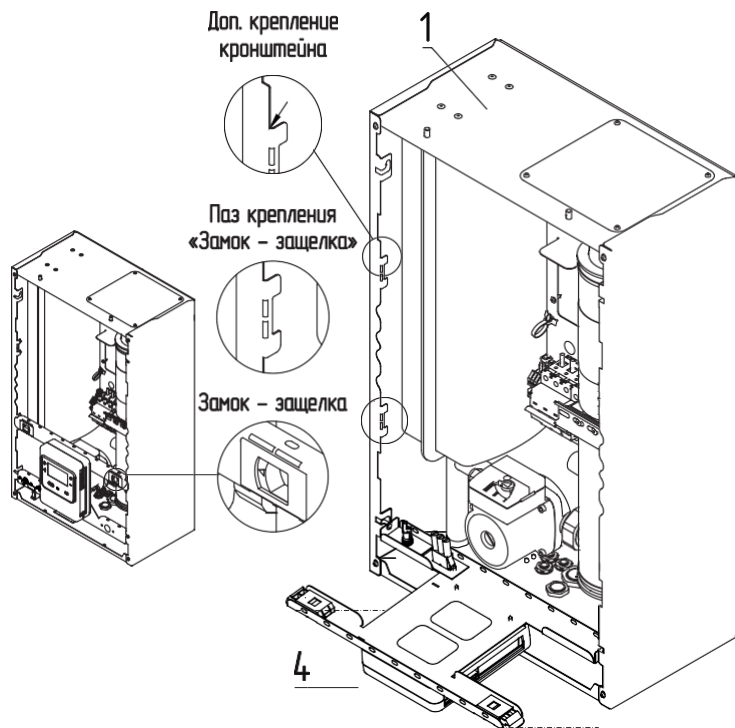
Рис.8 откидывание кронштейна
