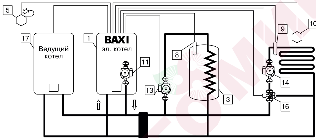
Схема 3.3 Контур ГВС и контур трехходового смесительного клапана в режиме теплого пола.
