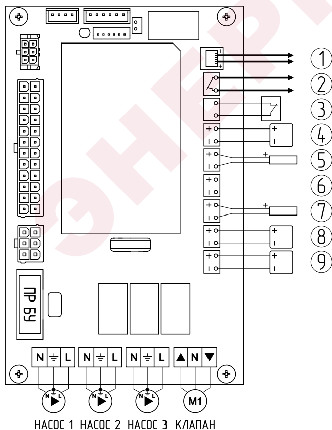
Рис.5 Схема подключения котла
