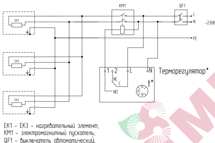
Рис.4. Обогреватель ВИН-APL-2.0-М
