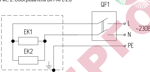
Рис. 2. Обогреватель ВИН-APL-2.0
