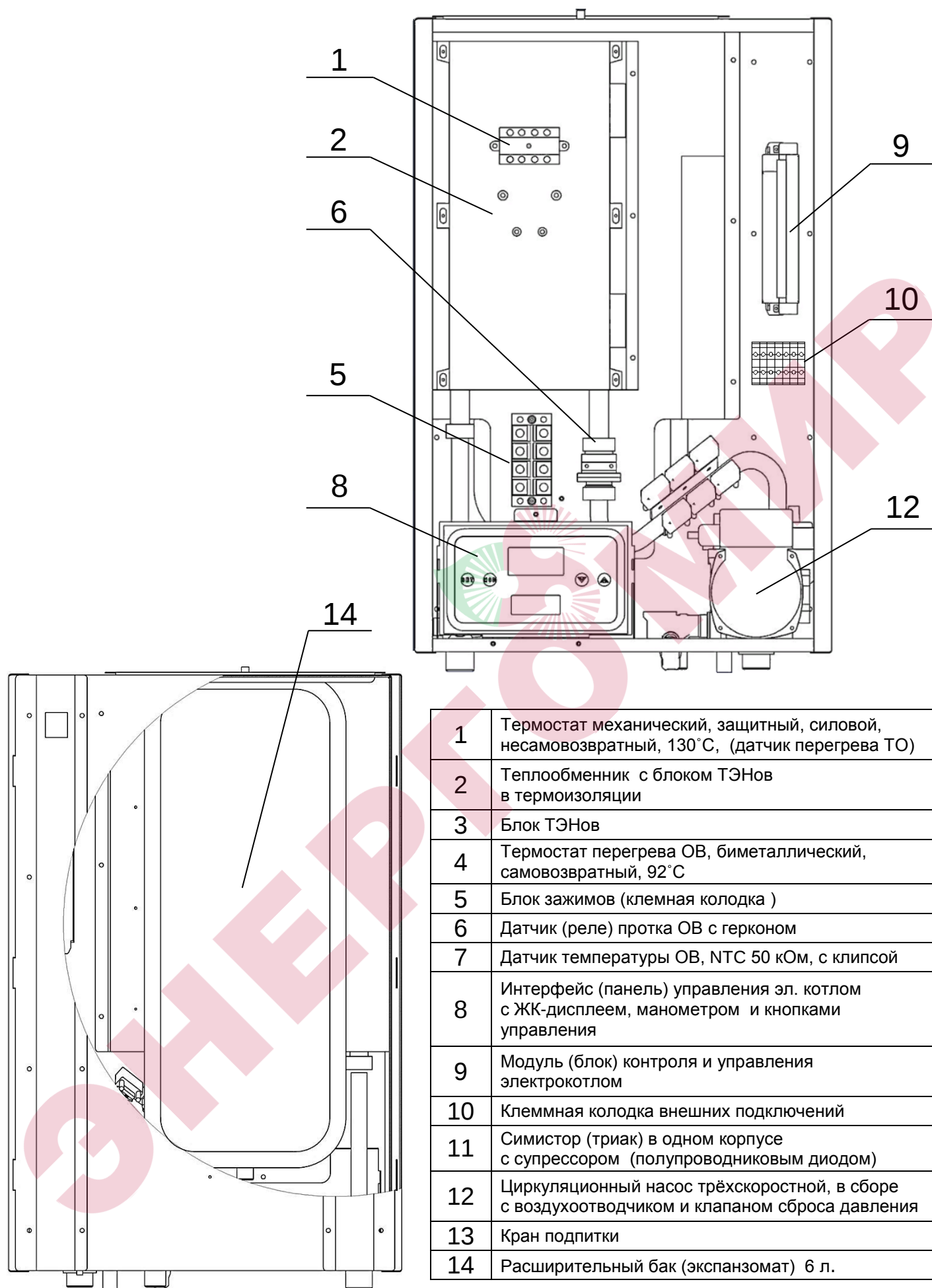
Рис. 2 Внутренне устройство
