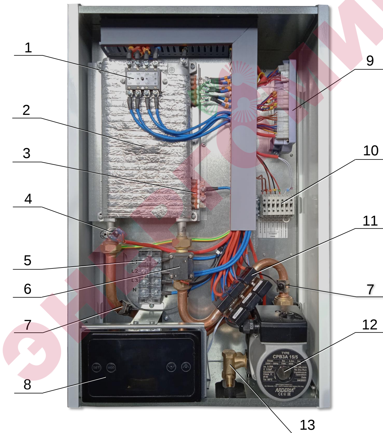
Рис. 1 Общий вид
