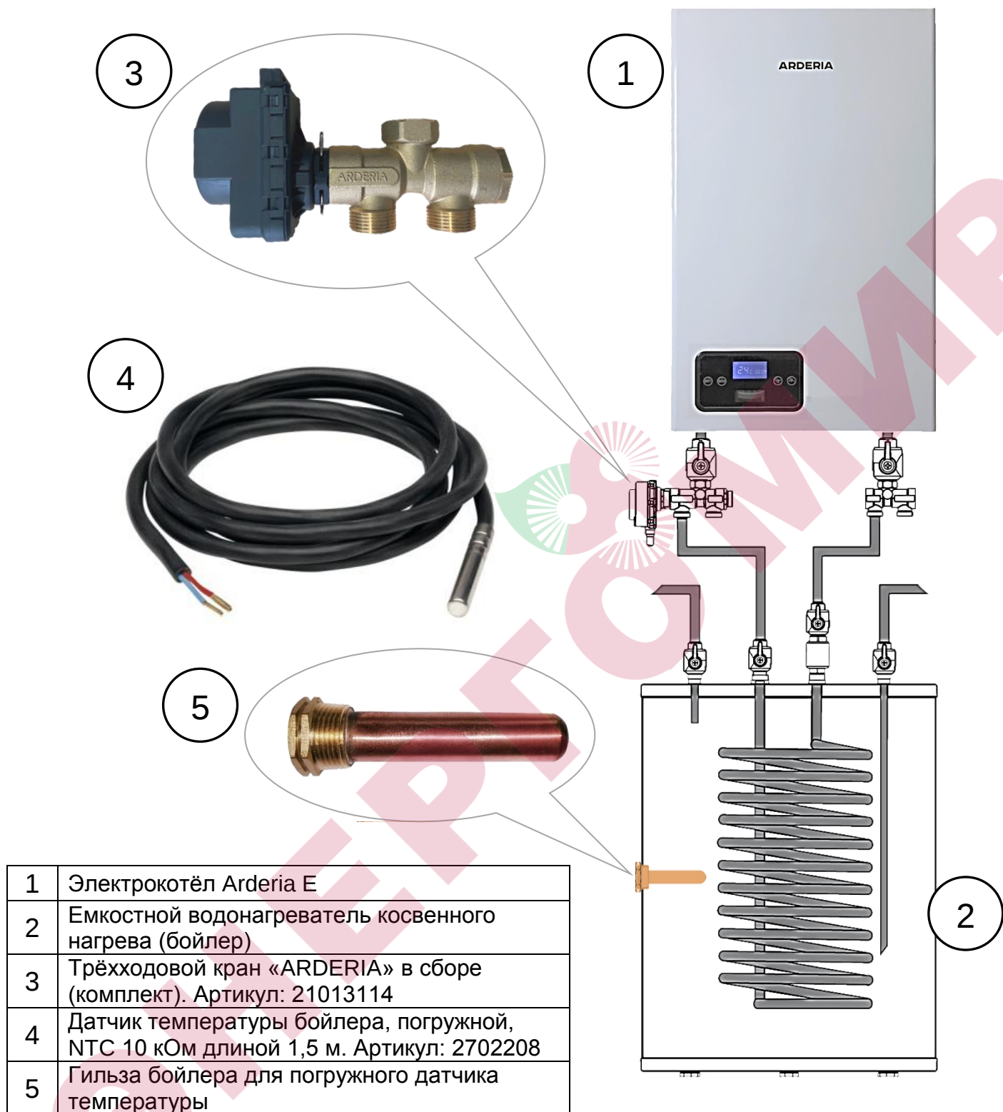
Рис. 22 Принципиальная монтажная схема подключения электрокотла к емкостному водонагревателю косвенного нагрева (бойлеру)
