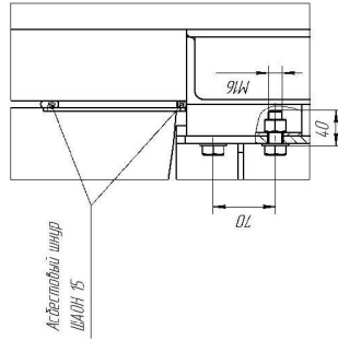
Д (Крепление стоек)
