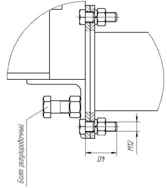
Д (Крепление стоек)
