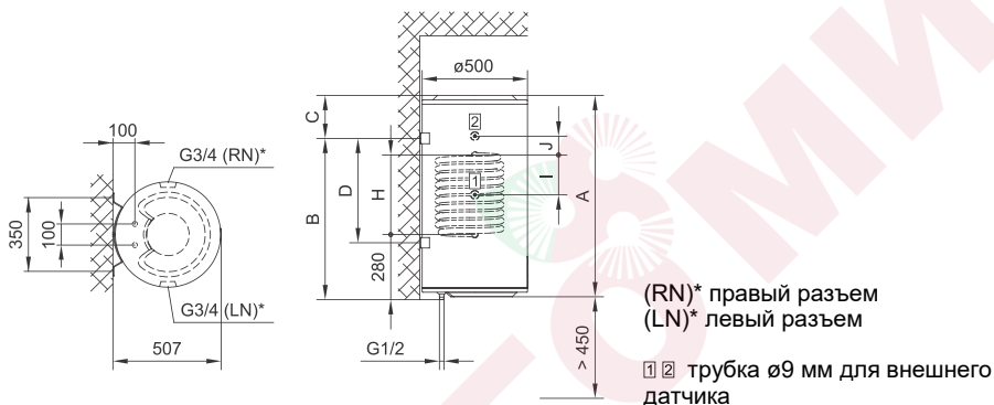
Рис. 1: Монтаж на стену в вертикальном положении
