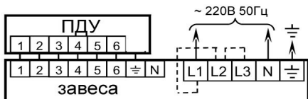
Рис. 3. Схемы подключения завес к электросети и пульту управления
