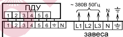
Рис. 3. Схемы подключения завес к электросети и пульту управления
