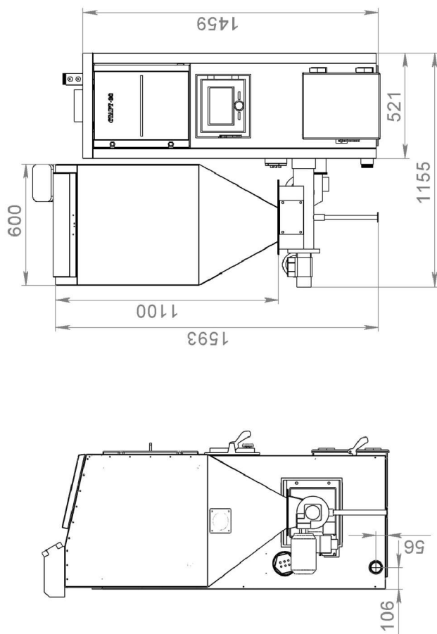
Пеллетный котел "СТАРТ-30-GR-V1", бункер 300 литров
