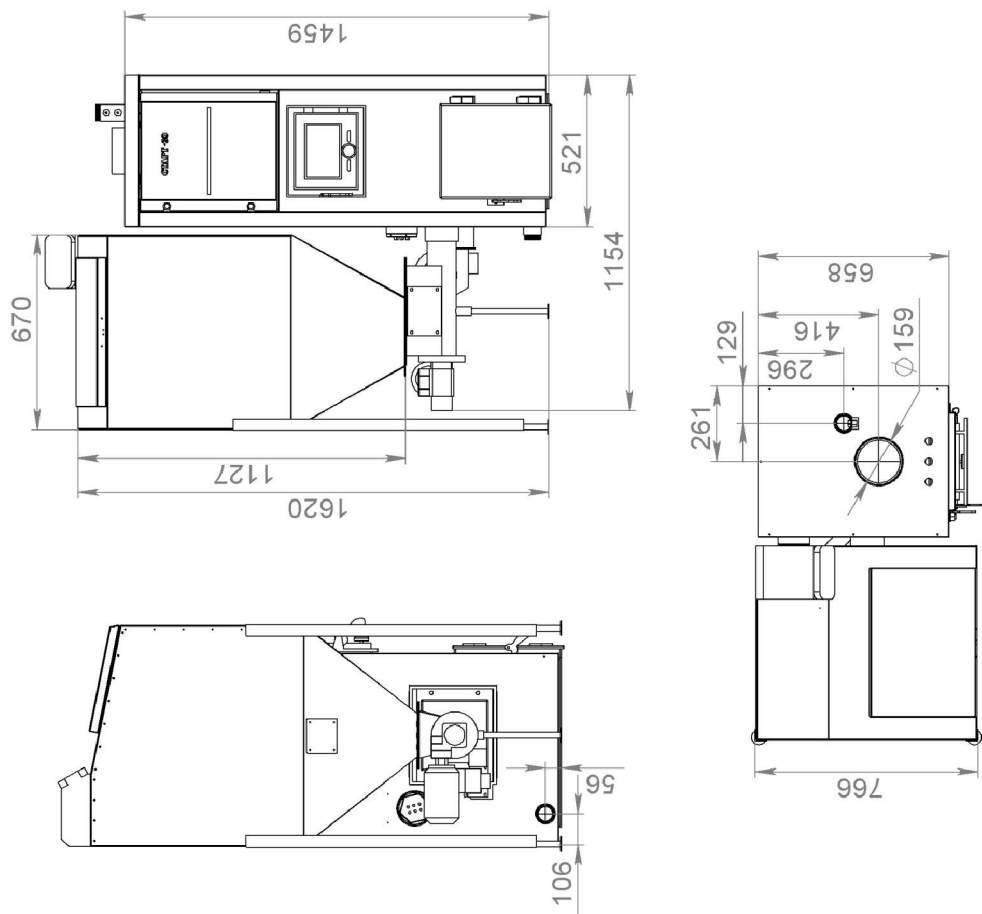
Пеллетный котел "СТАРТ-30-GR-V1", бункер 400 литров
