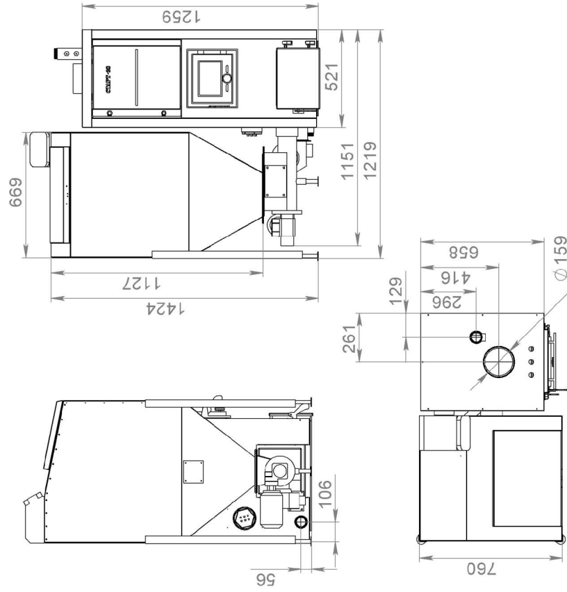
Пеллетный котел "СТАРТ-30-GR" (с бункером 400 литров)
