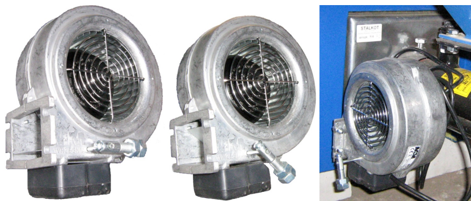
Рисунок 6 – Регулировка положения заслонки вентилятора
