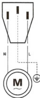
Рисунок 8 – Схема подключения проводов циркуляционного насоса
