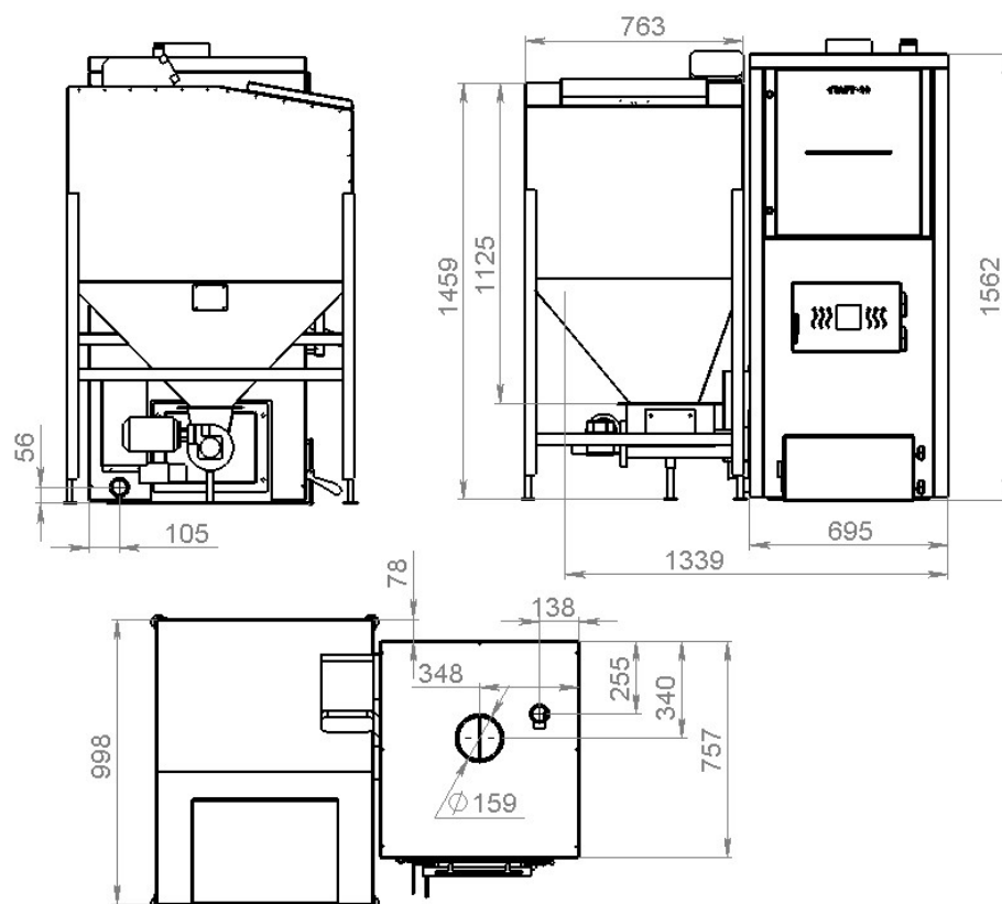
Пеллетный котел "СТАРТ-50-GR" (с бункером 600 литров)
