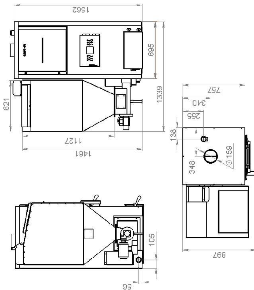
Пеллетный котел "СТАРТ-50-GR" (с бункером 600 литров)
