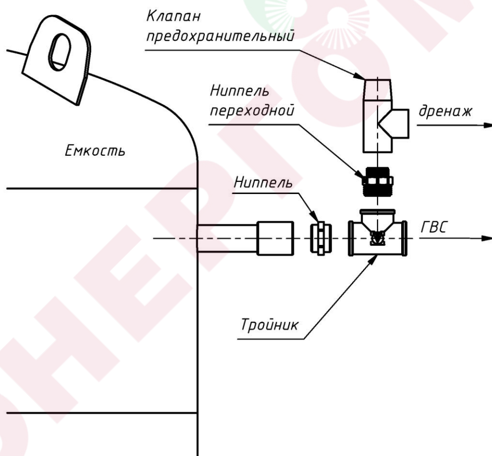
Схема сборки и установки предохранительного клапана
