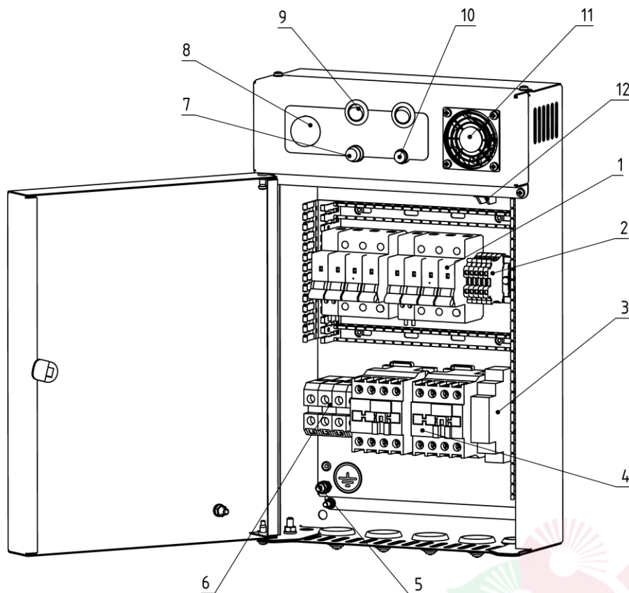
Рис. 2. Панель шкафа управления (опция) 5 – 40 кВт.
