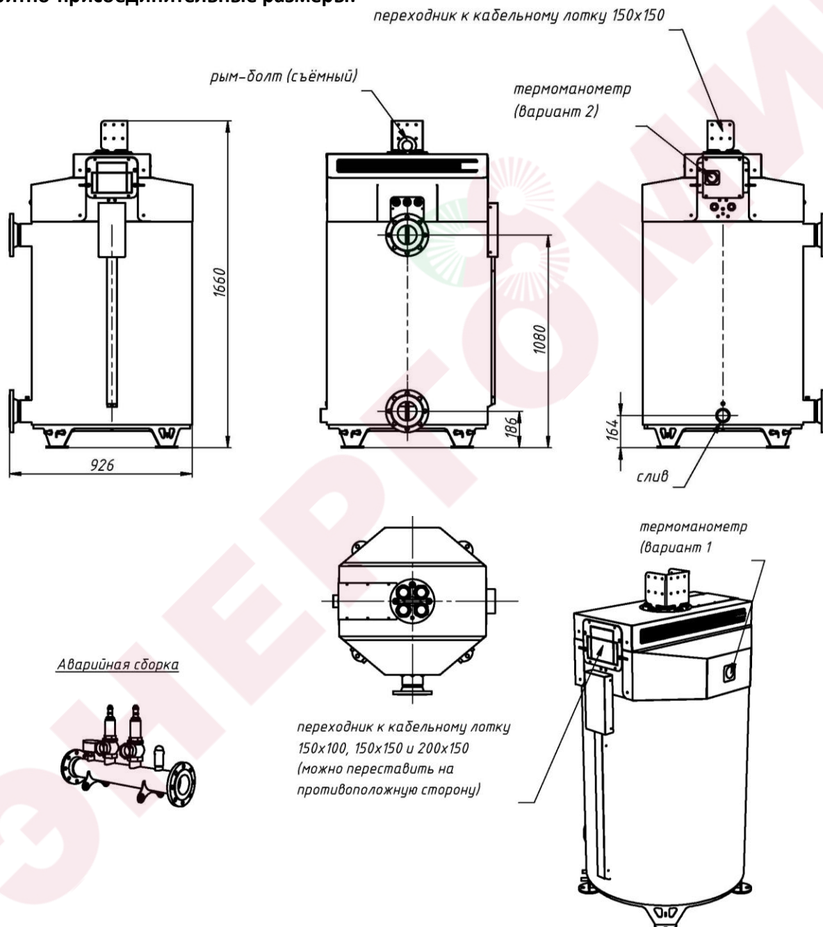
Бак котла, на примере КЭН-П 40 (Рис. 1)
