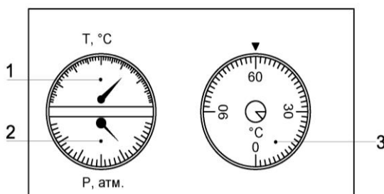
1 – Термометр, 2 – Манометр, 3 – Термоограничитель
