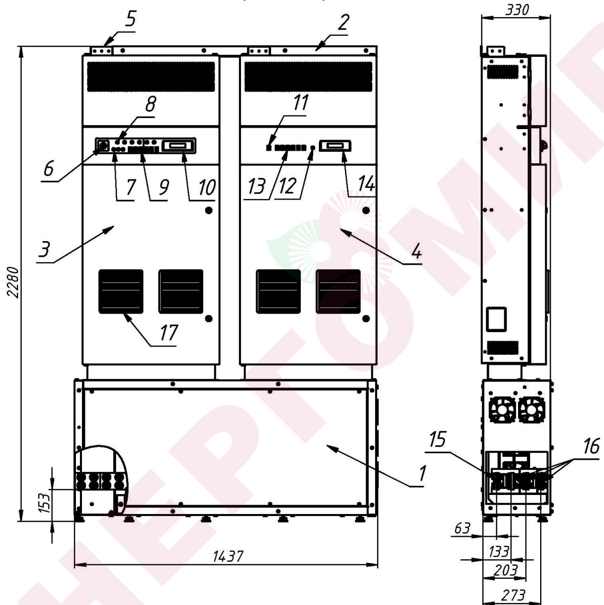
Шкаф автоматики и управления, на примере ШАУ 1000 кВт (Рис. 2)
