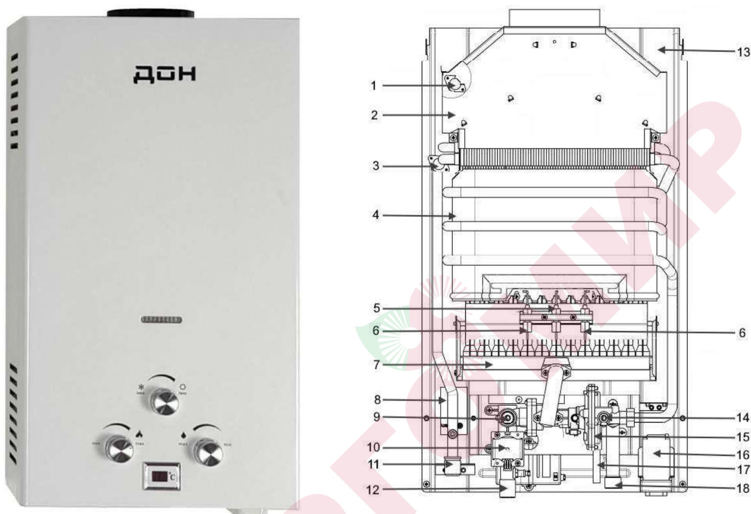
Рис. 1. Аппарат водонагревательный проточный газовый бытовой
