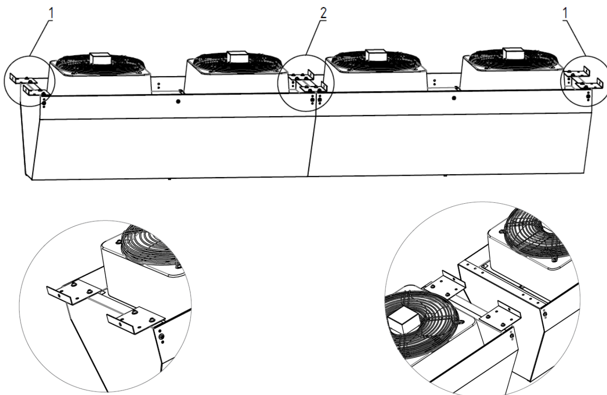
Рис. 1. Крепежные элементы завес
