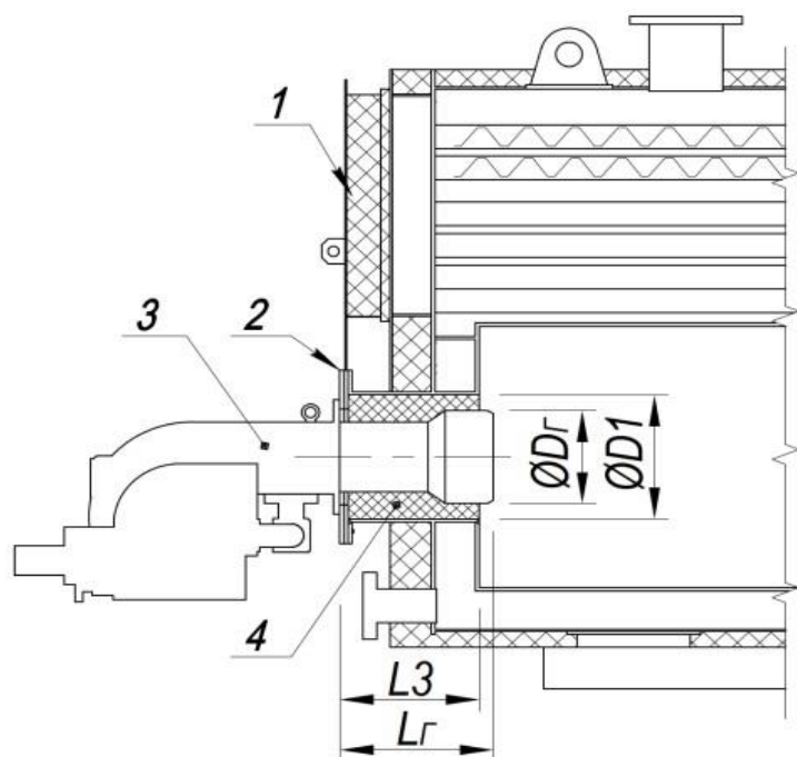
Рисунок 4. Установка горелки
