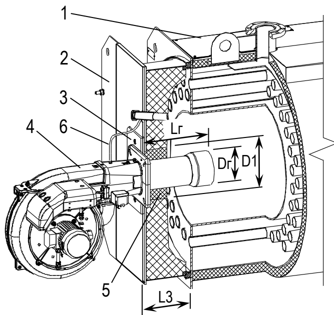
Рисунок 4. Установка горелки
