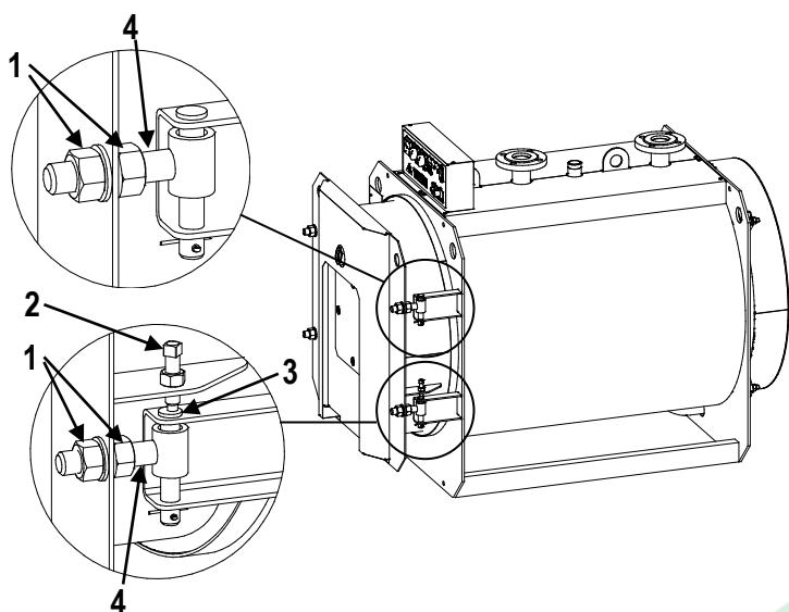
Рисунок 3.1 Петли передней двери топки котла
