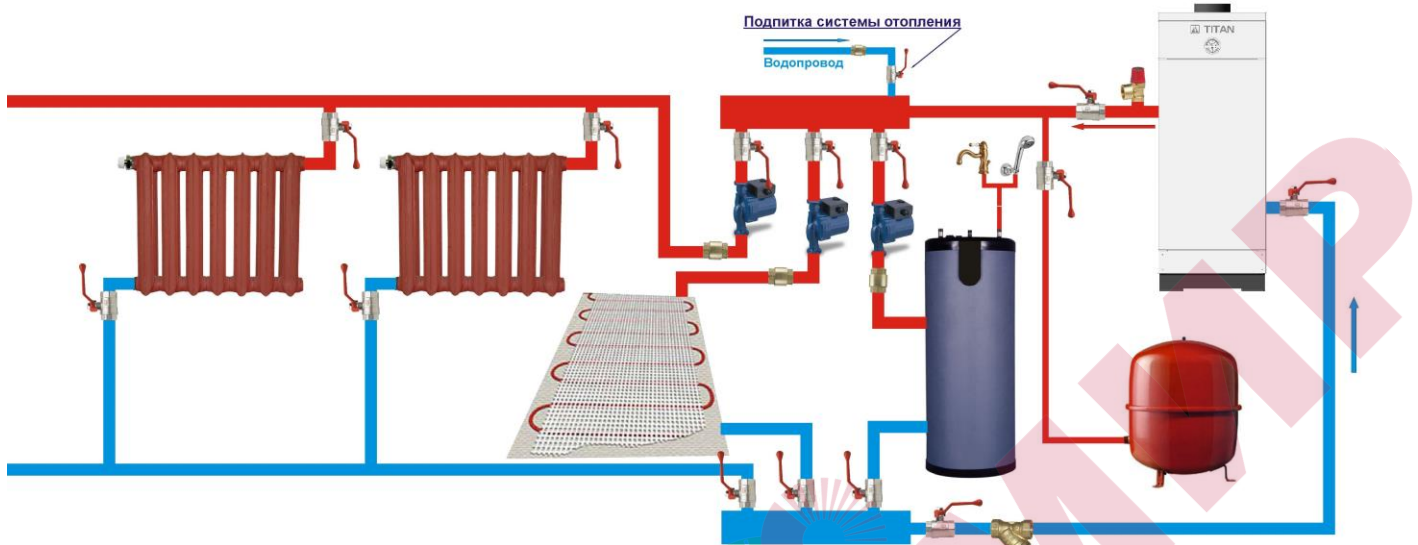
Рисунок 6. Схема подключения котла с общим коллектором
