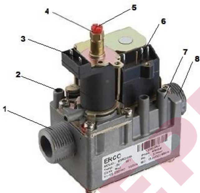
Рисунок 10. Газовый клапан котла. (показан со снятым защитным колпачком)
