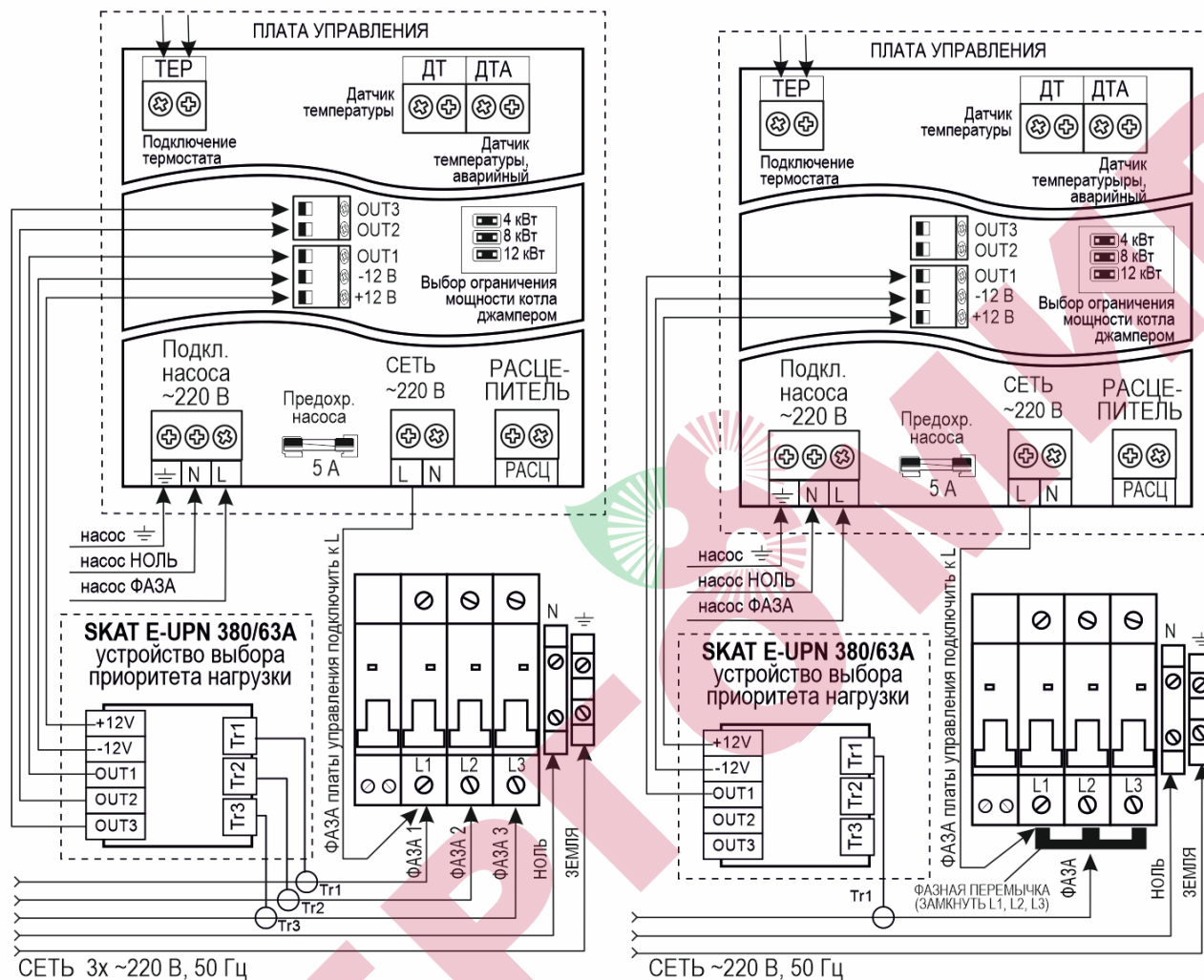
Схема подключения электрокотла к сетям ~220 В и 3x~220 В
