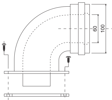
Рис. 14. Элементы присоединения коаксиальной системы дымоудаления к котлу.
