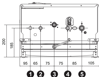
Рис. 5. Присоединительные размеры котлов
