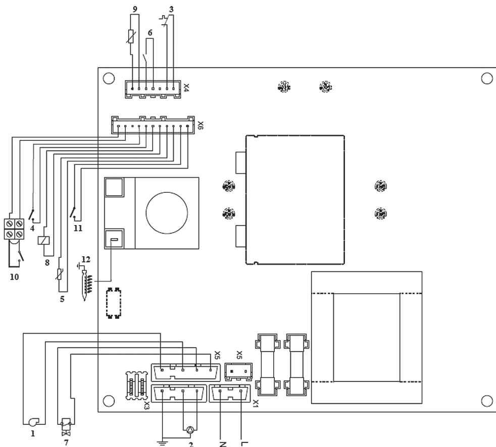
Рис.7. Принципиальная электрическая схема
