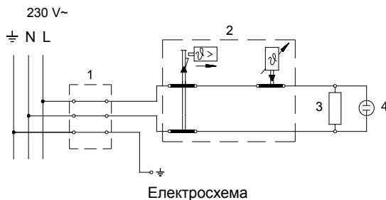
Електросхема
