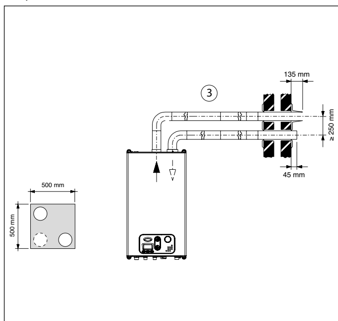
Рис. 11 Пример системы воздухозабора / дымоотвода
