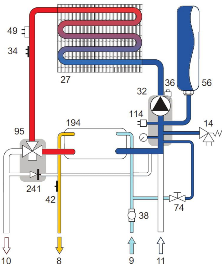
рис. 18 – Контур ГВС
