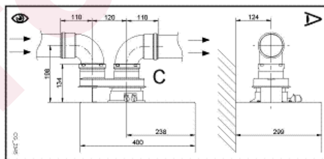
(С) – разделительный комплект
