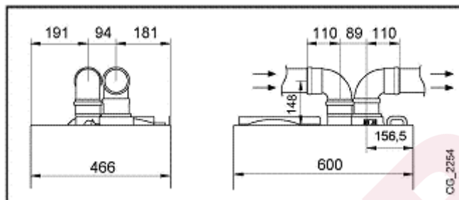
(А) – труба подачи воздуха (В) – труба выводов продуктов сгорания
