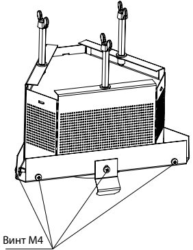
Рис. 11 Установка винтов на дожигатель
