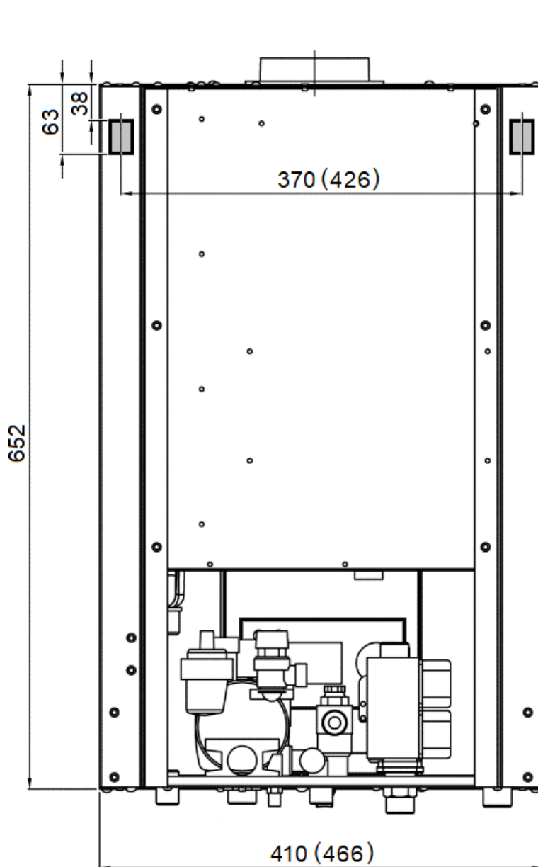
Рис. 6 Габаритные размеры моделей B21 / B24, D21 / D24 и S24 (в скобках указаны габаритные размеры моделей D28 / D32 / D40 и S28 / S32 / S40)
