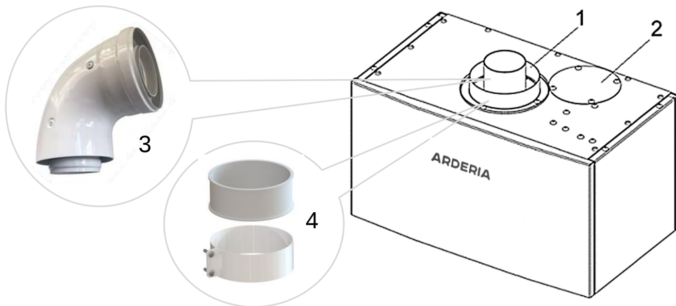
Рис. 25 Присоединительные элементы системы дымоудаления котлов Arderia
