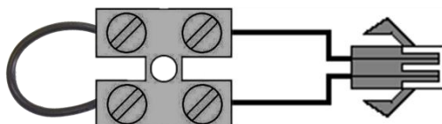
Рис. 45 Подключение перемычки (шунта) к клеммной колодке
