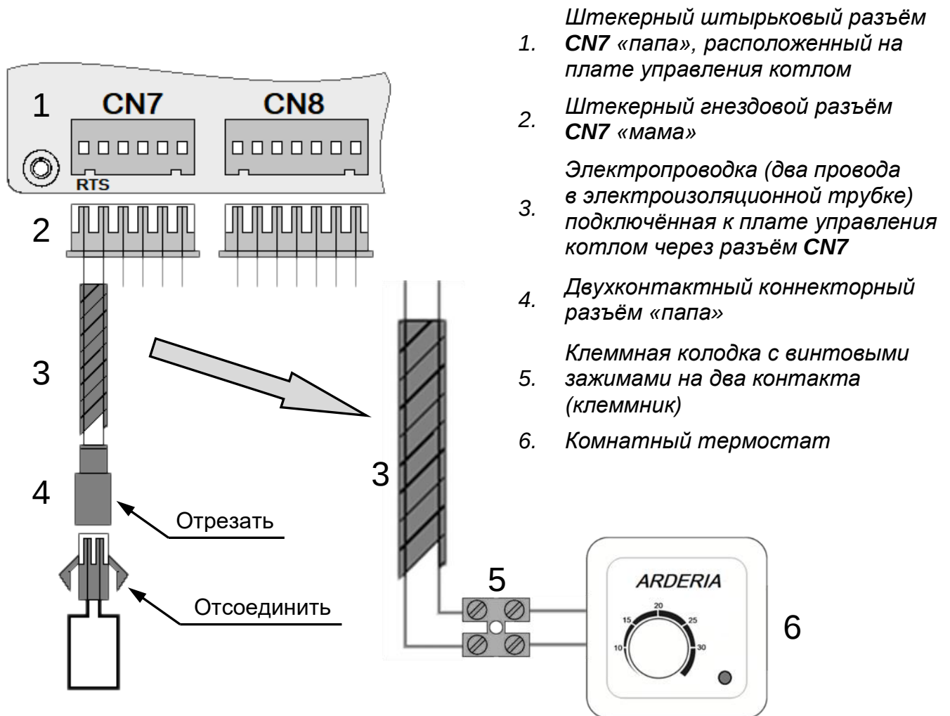
Рис. 46 Принципиальная схема подключения комнатного термостата непосредственно к электропроводке (двум проводам в электроизоляционной трубке) присоединённой к плате управления котлом через разъём CN7
