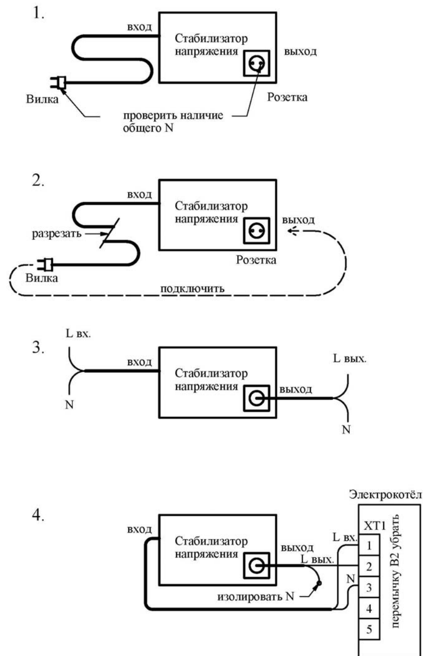
16. Схема подключения стабилизатора напряжения к электрическому котлу Рис. 9
