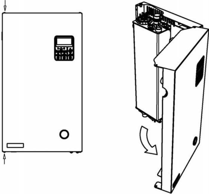
Рис. 2 и Рис. 3 Винты, откручиваемые для открытия крышки кожуха
